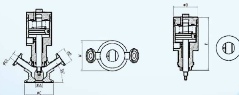
Fig. 2. Dimensions - actuator
